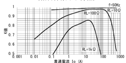
〔結合係数 (K) 特性〕
