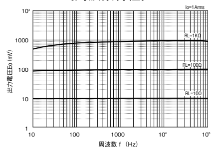
〔周波数特性〕
